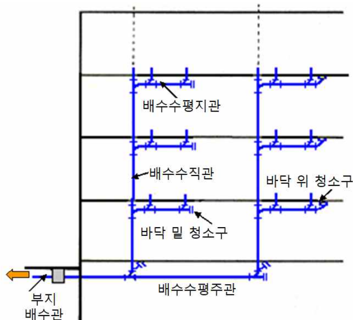
(a) 배수수평지관, 배수수직관, 배수수평주관
