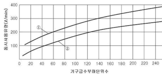
(b) 동시사용유량 (일부확대)
