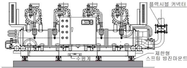
-장비 하부 스프링 방진스프링 마운트 설치 도면 및 설치 모습-
