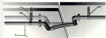
-수직변위 발생 시 제어모습-
